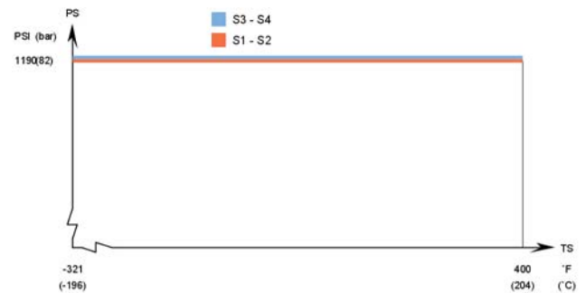
CBXP27 – Gráfico de presión/temperatura con homologación UL
