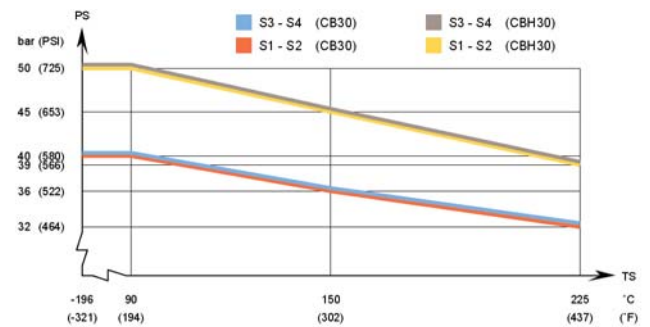
CB30 – Gráfico de presión/temperatura con homologación UL
