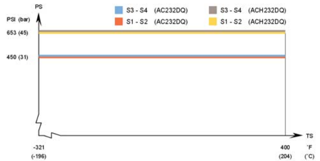
AC232DQ/ACH232DQ – Gráfico de presión/temperatura con homologación UL
