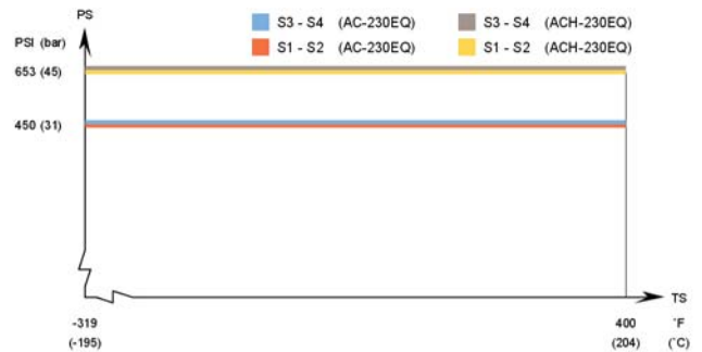
AC230EQ/ACH230EQ – Gráfico de presión/temperatura con homologación UL
