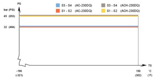
AC230DQ/ACH230DQ – Gráfico de presión/temperatura con homologación UL
